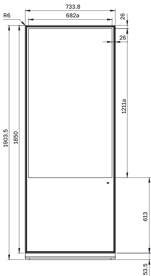
СХЕМА ДИСПЛЕЯ (ВИД СПЕРЕДИ)
